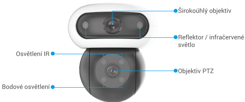
Pohled zepředu
